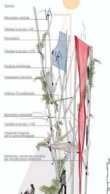
Sezione
