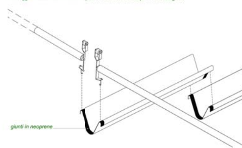
3A montaggio a secco delle canaline per la raccolta delle acque meteorologiche
